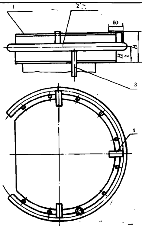
图 Q7 旋风分离器立式圆型顶帽出口的圆环式蒸汽取样器及安装示意图
